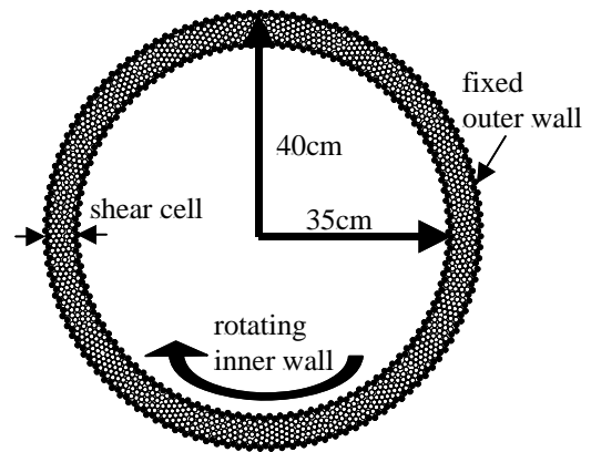
Fig. 2 DEM数値実験で用いた境界条件
