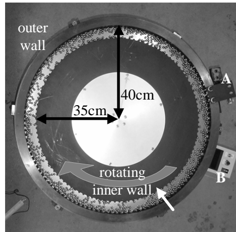
Fig.1 粒状体高速せん断実験装置(モデル実験)
