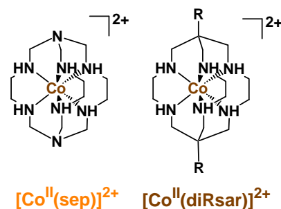
図2 籠状金属錯体
