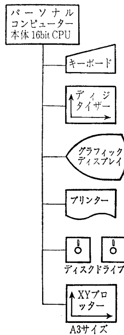
図-2 パソコンを用いたハードウェア構成の例 9)
