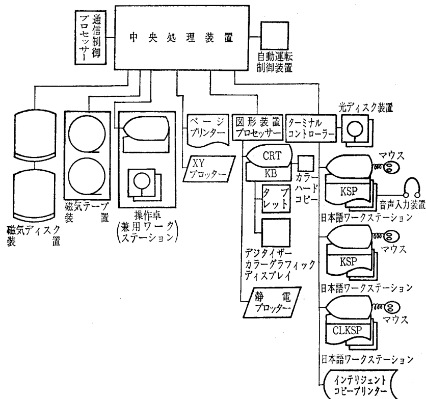
図-1 汎用機を用いたハードウェア構成の例(文献8)を一部修正)
