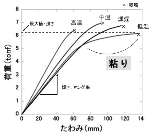
図3 乾燥温度とたわみ (17)
