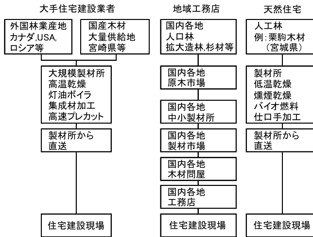
図1 森林から住宅建設現場までの木材の供給経路比較
