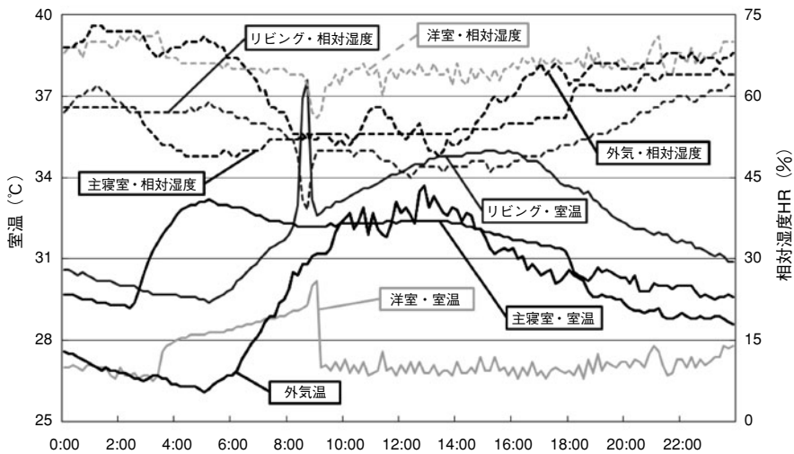
図4 天然住宅 室内環境実測例 (Y邸・目黒区) 2011年7月17日
