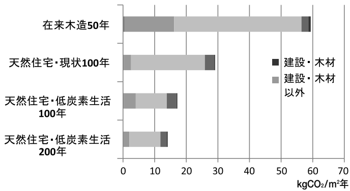
図8 天然住宅 LCCO 2 想定寿命別比較
