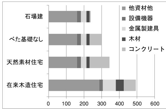
図6 建設誘発 CO 2 排出量 kgCO 2 /m 2
