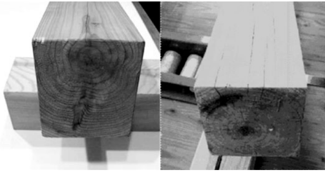
写真3 低温乾燥材(左)と高温乾燥材(右) (18)
