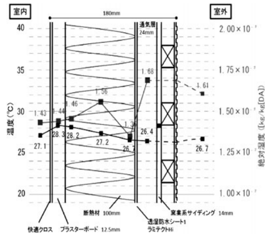
図5 天然住宅 壁対温度湿度傾斜・実測結果(Y邸・目黒区) 2011年7月17日
