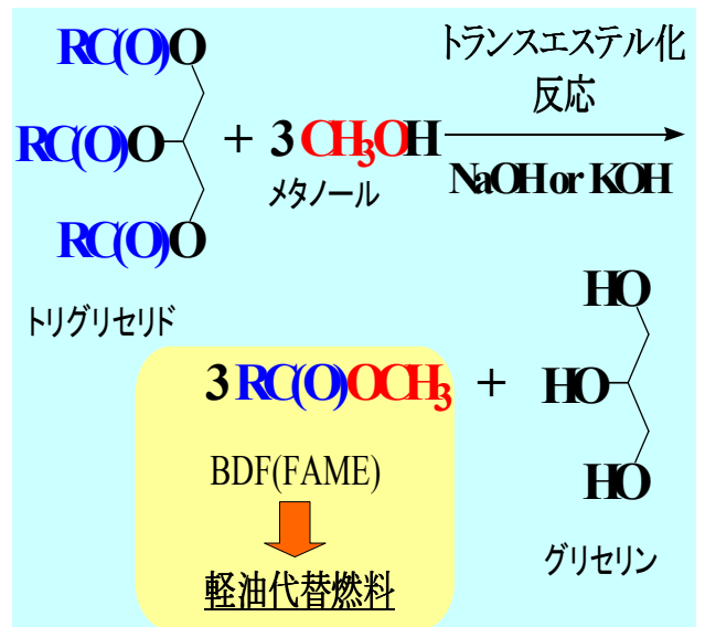
BDF:バイオディーゼル燃料の合成
